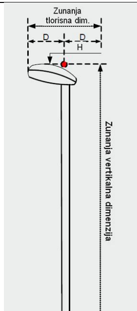
Svetilo na drogu javne razsvetljave
