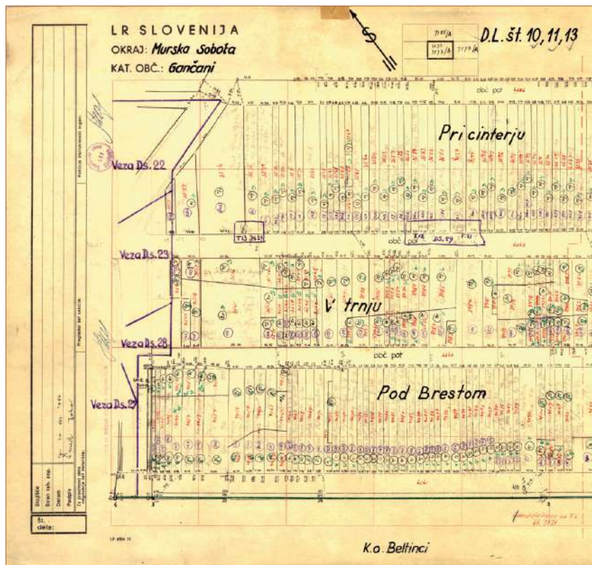
Slika 5.2.4.2: Primer terenske skice enoslikovne fotogrametrične izmere k. o. 129 Gančani z merjenimi širinami parcel za skupno uporabo s fotokscami.
