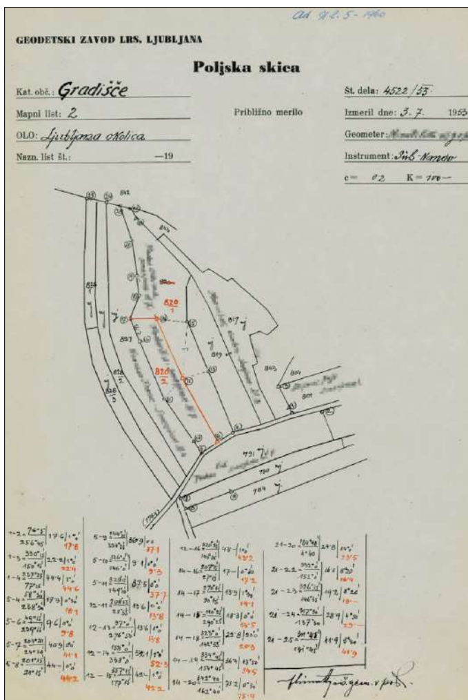
Slika 2.5.13: Skica izmere k. o. 1710 Gradišče iz leta 1953, kjer se je meritev opravila z busolnim teodolitom na preskok.
