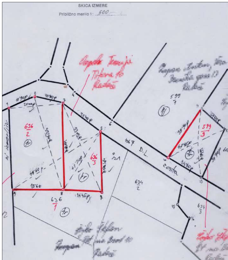
Slika 2.5.17: Skica izmere k. o. 1866 Hote- mež v približnem merilu 1 : 500, parcelacijski načrt v M 1 : 2880 in kartiranje z upoštevan- jem skrčka (elaborat iz leta 1989, zamejničen- je ceste le z ene strani).
