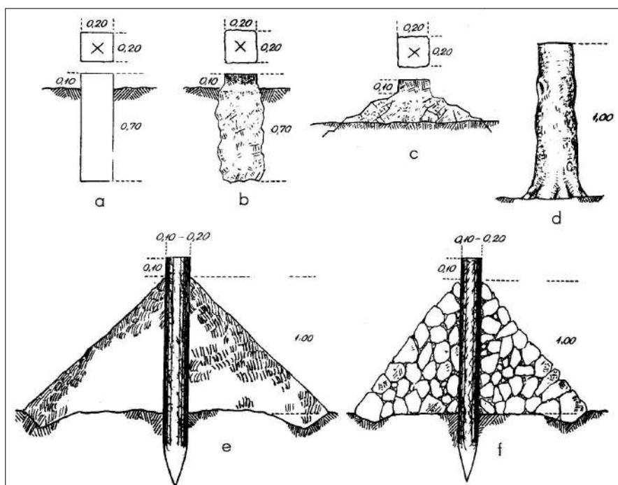
Slika 5.2.1.1: Možne vrste označitve zamejničenja mej k. o. s trajnimi znamenji predpisanih dimenzij – a) betonski kamen, b) naravni kamen z obklesano glavo c) urezana oznaka v skalo, d) prisekano deblo, e) lesen kol v humki zemljine in f) lesen kol v humki zloženega kamenja.
