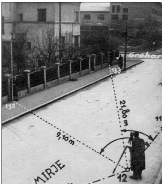
Slika 5.2.3.1: Prikaz načina polarne snemanja. Vir: Arhiv GURS
