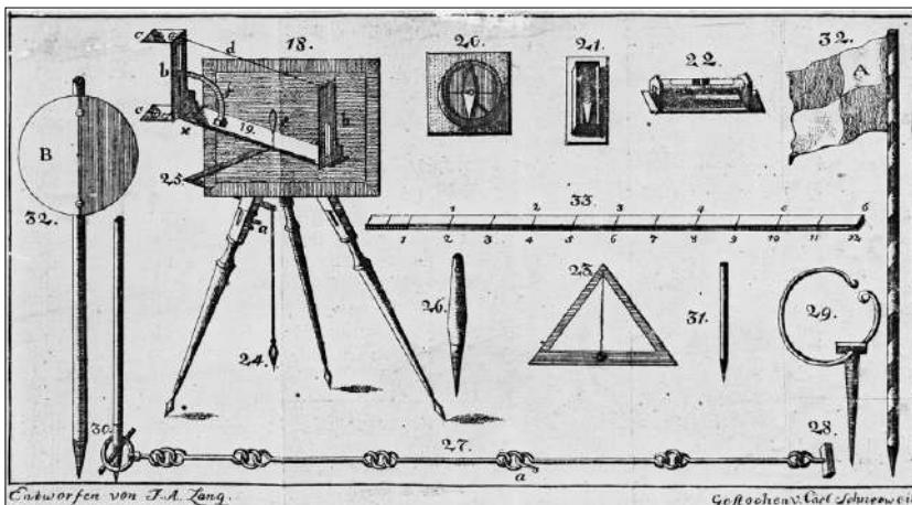
Slika 2.2.5: Obvezna merska oprema za detajlno izmero v prvi polovici 19. stoletja in pozneje tudi pri reambulaciji grafičnega katastra (merilna mizica, vodna tehtnica, dioptrsko ravnilo, svinčnica, 10 col dolga merska veriga in risalni pribor).
